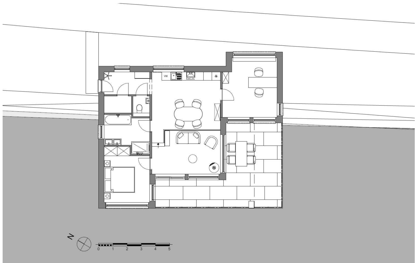
Grondplan / ArchiCAD
