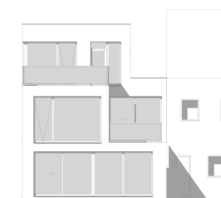
ACHTERGEVEL
