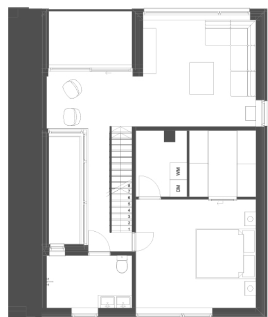
NIVEAU 1
