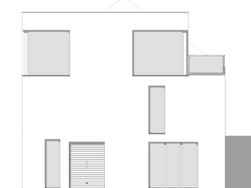
RECHTERZIJGEVEL
