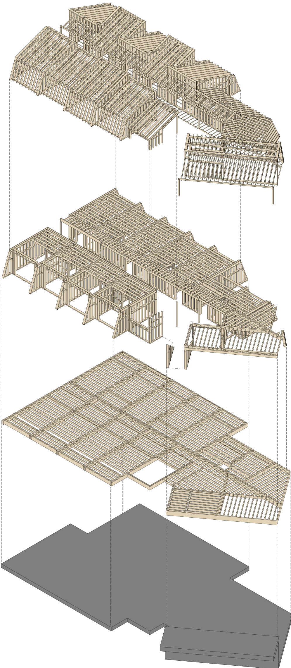
Axonometie van constructief model / archicad
