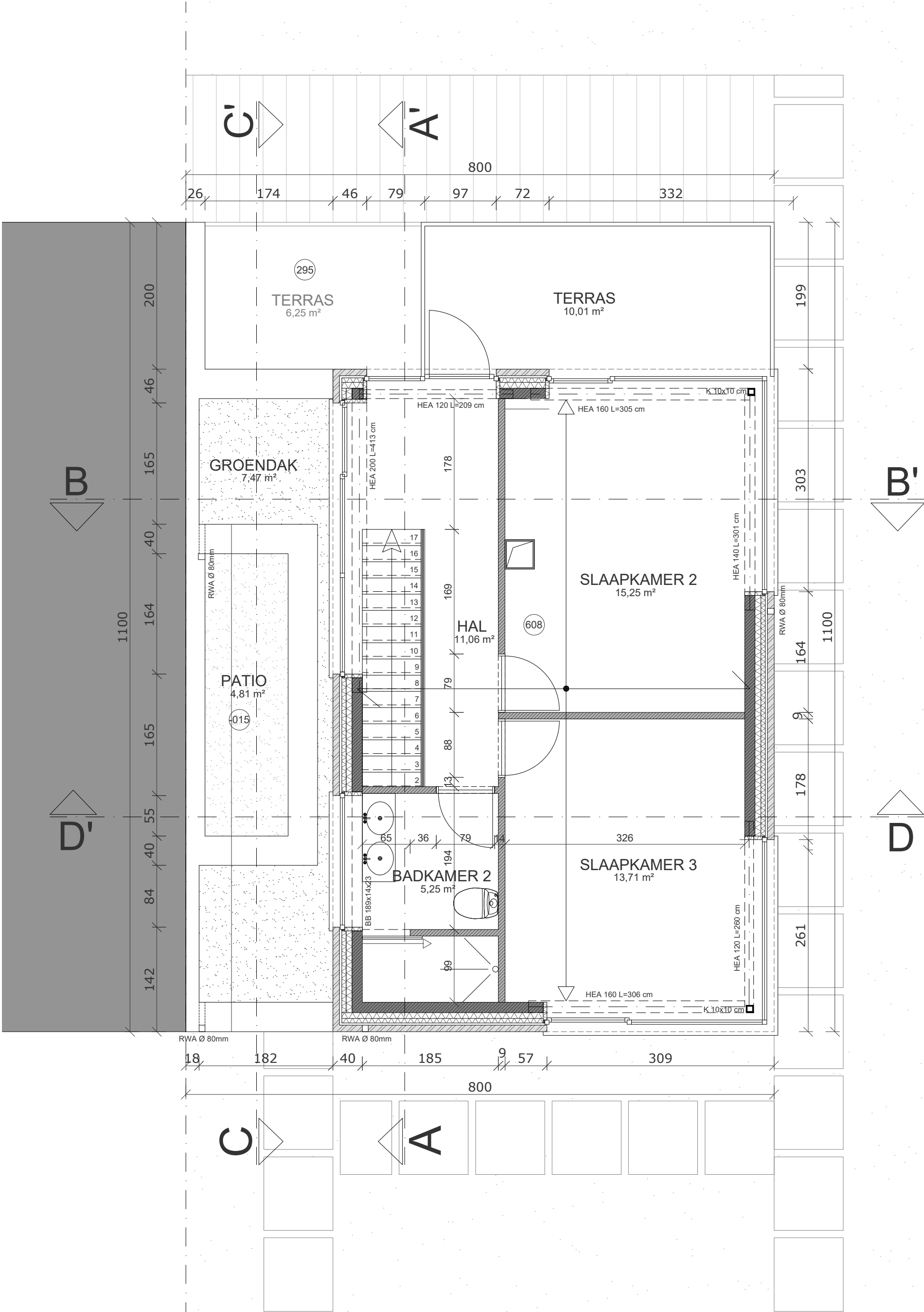
GRONDPLAN NIVEAU 2
