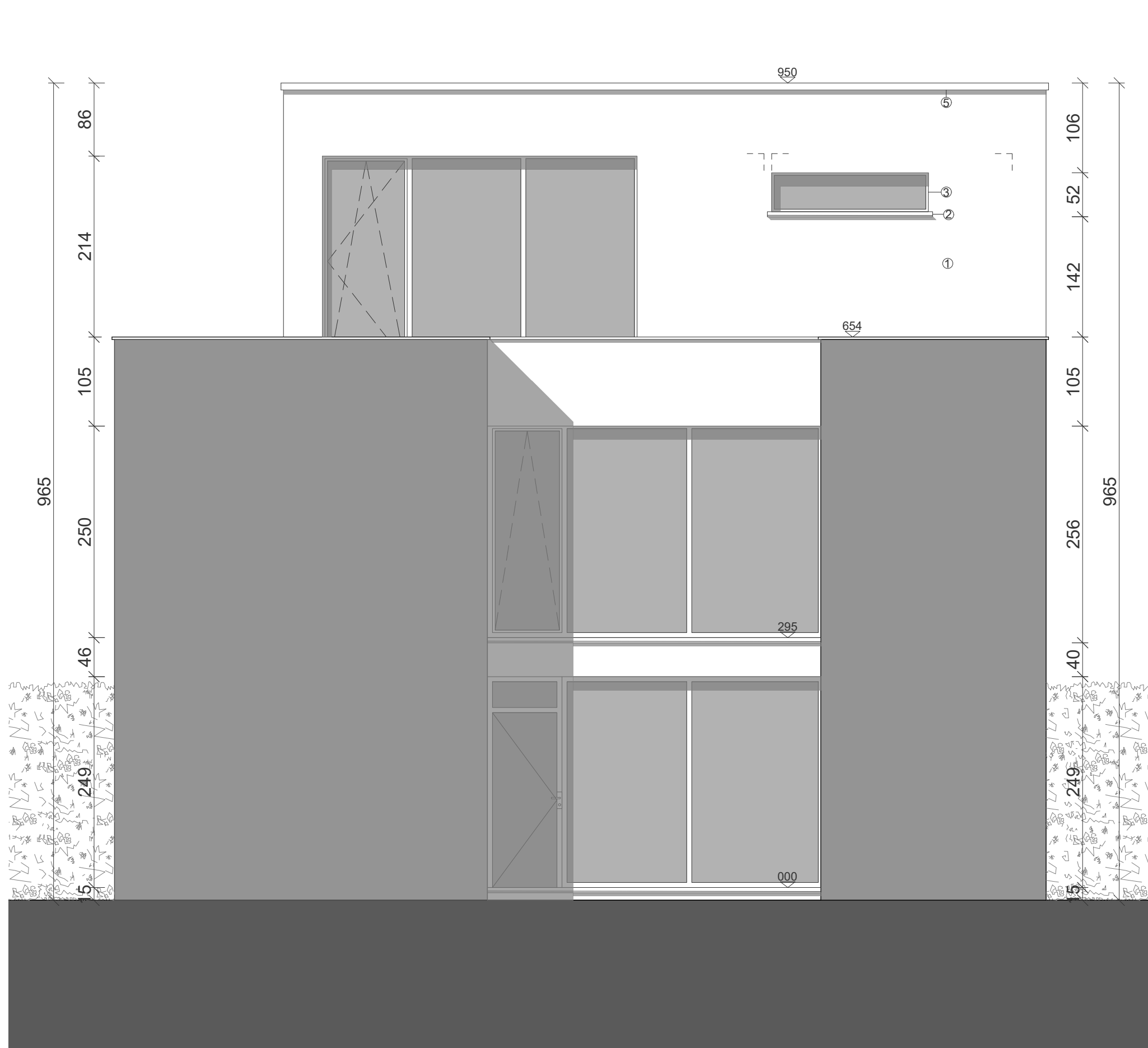
LINKERZIJGEVEL
