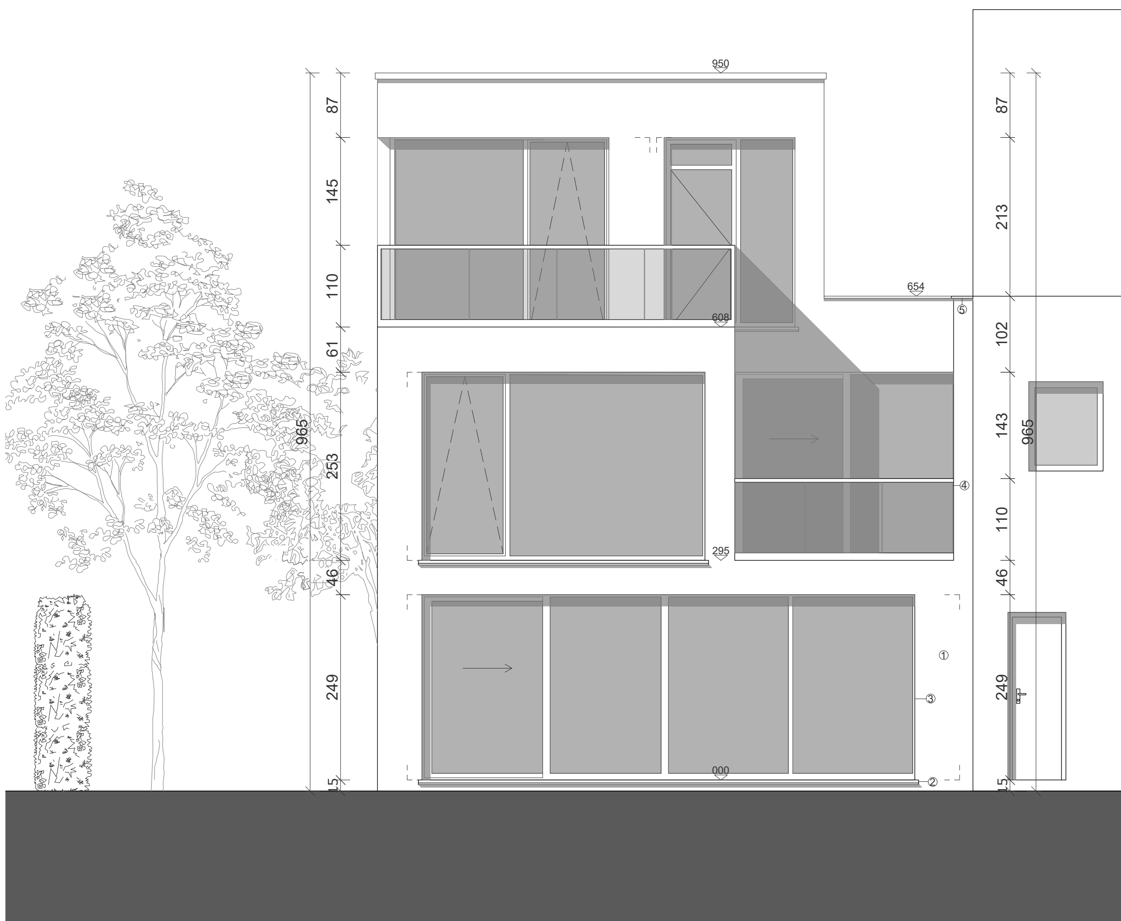
ACHTERGEVEL
