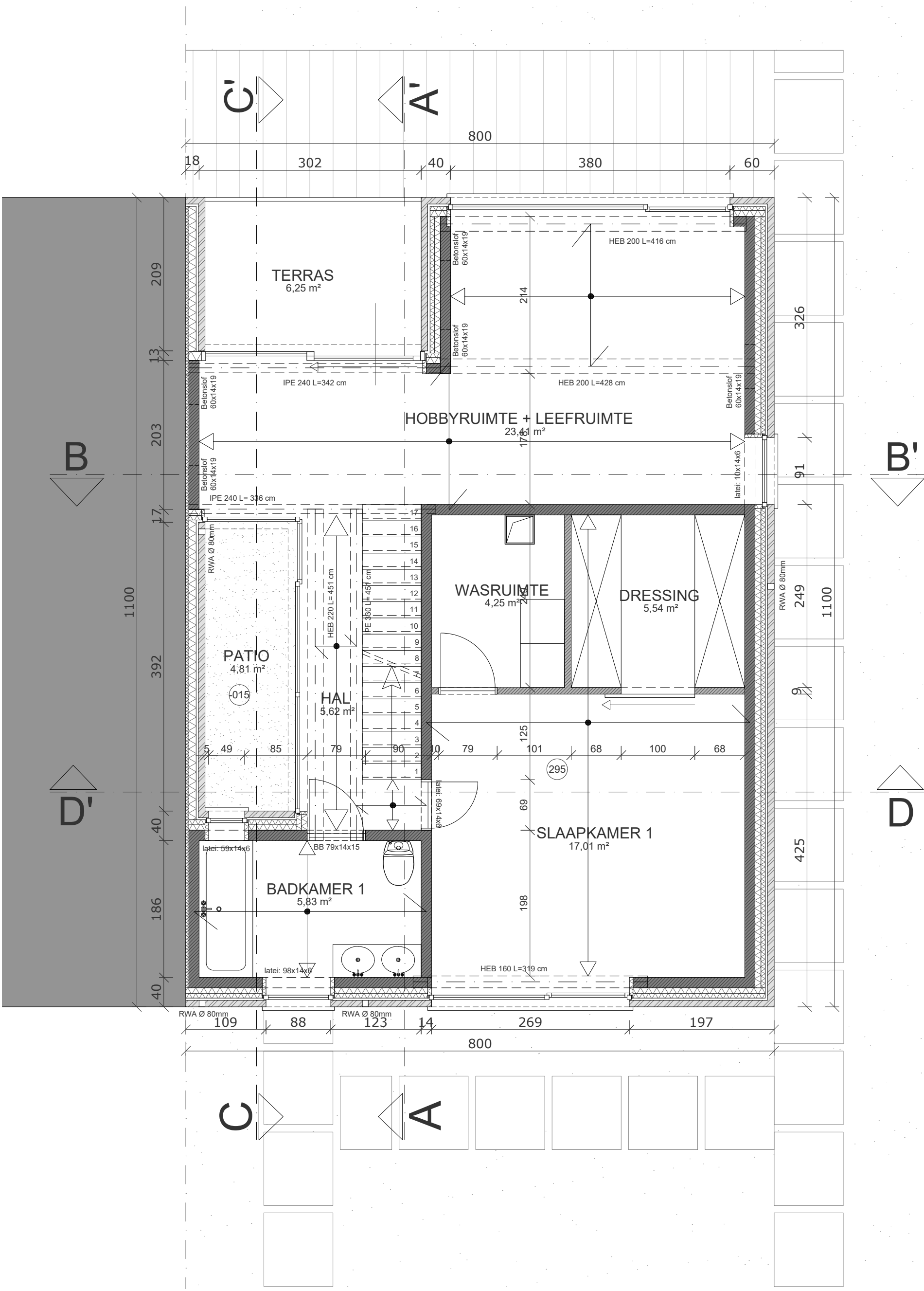
GRONDPLAN NIVEAU 1
