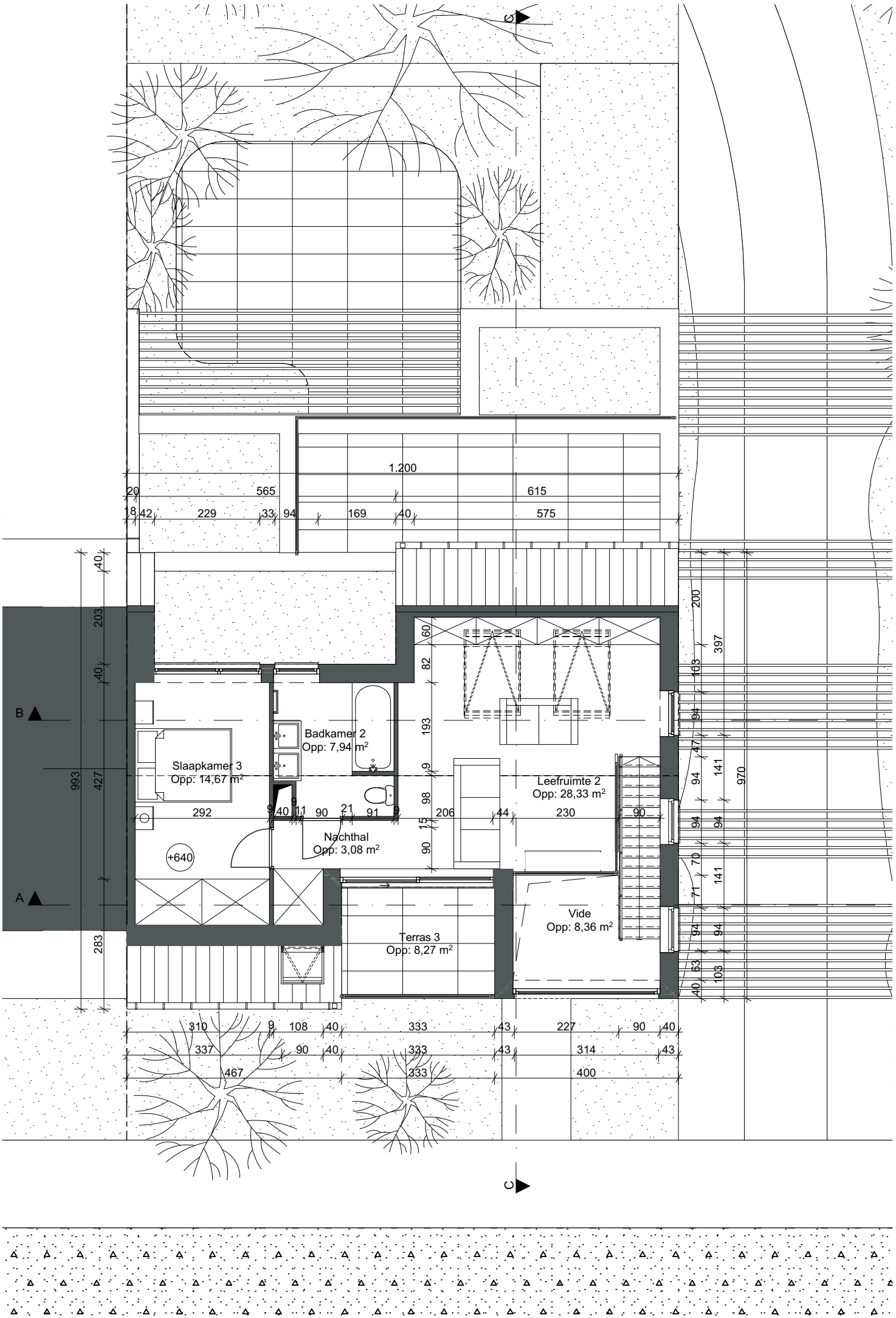
Grondplan +2 (Schaal 1:100)
